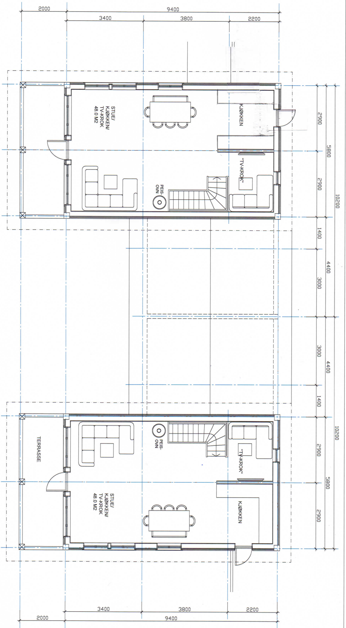
PLAN HOVEDTASJE 1:100 BRUKSAREAL PR. ENHET: 48,0 M 2
