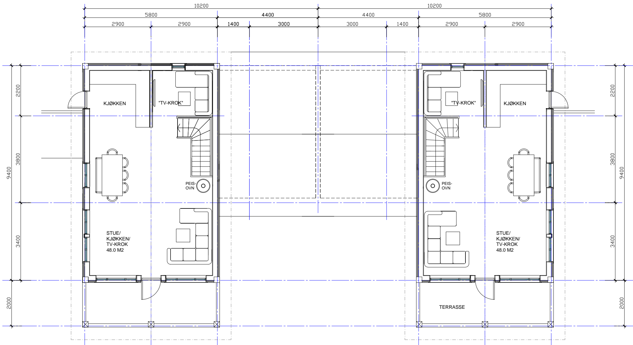
PLAN HØVEDETASJE 1:100 BRUKSAREAL PR. ENHET: 48.0 M2
