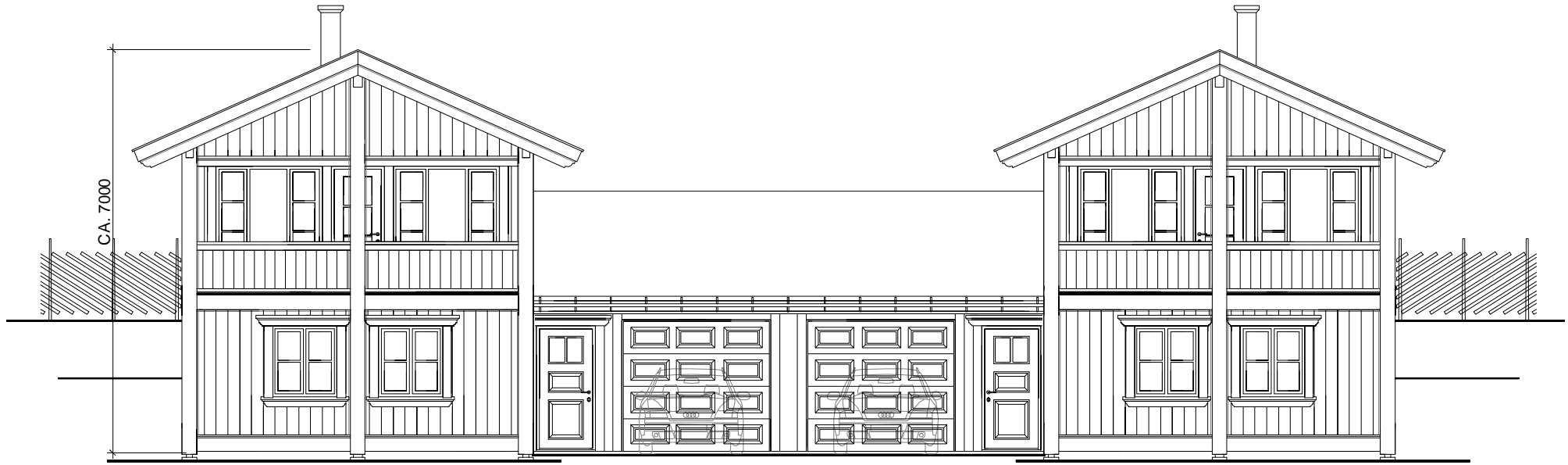
FASADE MOT NORD 1:100
